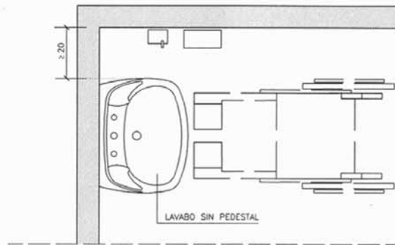
LAVABO ACCESIBLE
