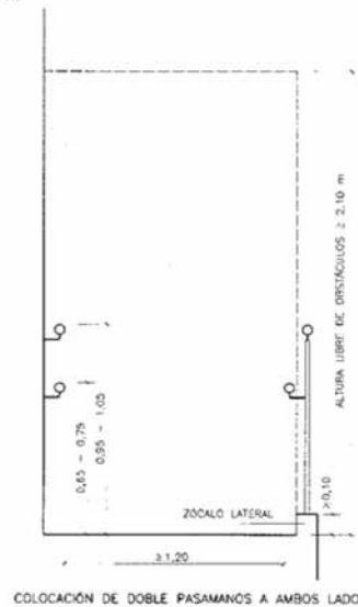
COLOCACIÓN DE DOBLE PASAMANOS A AMBOS LADOS
