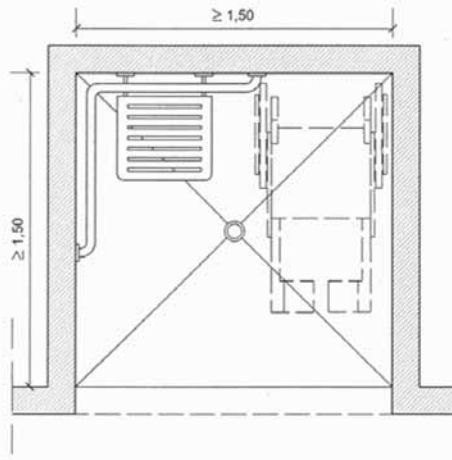
DUCHA ACCESIBLE EN RECINTO INDEPENDIENTE
